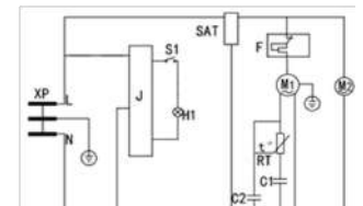
SD-206/336/416AELC/AEL XP - штепсель ашасы; SAT - Термостат; S1 - артқы жарық қосқышы; F - қорғаныс релесі; J - қуат қалқаны; M1 - Компрессор; H1 - ішкі подстветка; M2 - желдеткіш салқындату; RT - Стартер; C1 - іске қосу сыйымдылығы (жүзеге асыру кезінде); C2 - пайдалану сыйымдылығы (жүзеге асыру кезінде)
