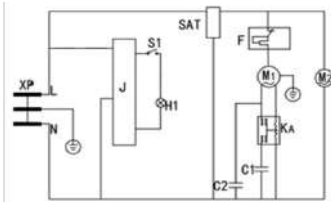
SD-516AELC/AEL XP – Штепсель ашасы; SAT – Термостат; S1 – Артқы жарық қосқышы; F – қорғаныс релесі; J - қорек қалқаны; M1 – Компрессор; KA – Стартер; H1 – ішкі подстветка; M2 – Салқындату желдеткіші; C1 – іске қосу сыйымдылығы (жүзеге асыру кезінде); C2 – Пайдалану сыйымдылығы (жүзеге асыру кезінде)
