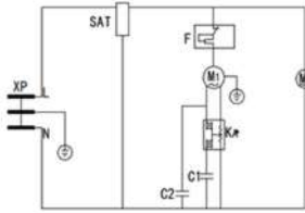
SD-516AEC/AE XP - Штепсельді айыр; SAT- Термостат; F – Қорғаныс релесі; M1-Компрессор; M2 - салқындату желдеткіші; KA-Стартер C1 - іске қосу сыйымдылығы (жүзеге асыру кезінде); C2 - пайдалану сыйымдылығы (жүзеге асыру кезінде)
