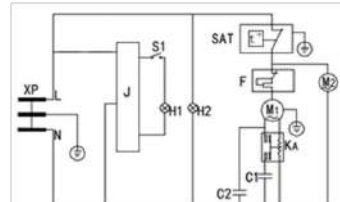
SD-516AMLC/AML XP - Штепсель ашасы; SAT - Термостат; J-қорек қалқаны; S1 - артқы жарық қосқышы; F - қорғаныс релесі; M1-Компрессор; H1 - ішкі подстветка; H2-қуат индикаторы; M2-салқындату желдеткіші; KA-Стартер; C1 - іске қосу сыйымдылығы (жүзеге асыру кезінде); C2-пайдалану сыйымдылығы (жүзеге асыру кезінде)
