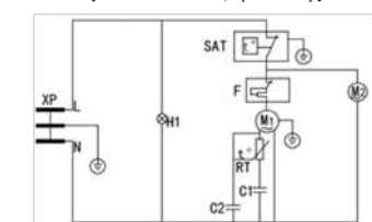
SD-206/336/416 AMC/AM XP - штепсель ашасы; SAT - Термостат; F - қорғаныс релесі; M1 - Компрессор; H1 - қуат индикаторы; M2 - салқындату желдеткіші; RT - Стартер; C1 - іске қосу сыйымдылығы (жүзеге асыру кезінде); C2 - пайдалану сыйымдылығы (жүзеге асыру кезінде)
