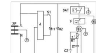
SD-206/336/416 AMLC/AML XP - штепсель ашасы; SAT - Термостат; S1 - артқы жарық қосқышы; F - қорғаныс релесі; J - қуат қалқаны; M1 - Компрессор; H1 - ішкі подстветка; H2 - қуат индикаторы; M2 - салқындату желдеткіші; RT - Стартер; C1 - іске қосу сыйымдылығы (жүзеге асыру кезінде); C2 - пайдалану сыйымдылығы (жүзеге асыру кезінде)
