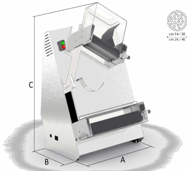
Рис. 2.7.1. – Тестораскаточная машина для пиццы SPR 30 / SPR 40
